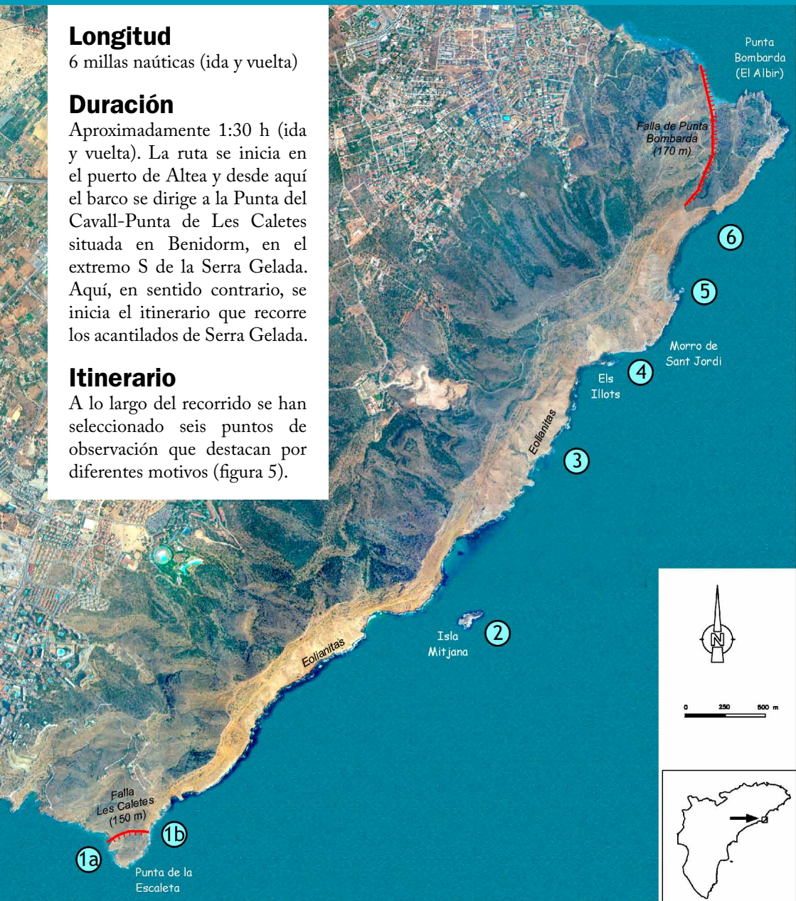
figura 5 - Fotografía aérea de Serra Gelada con la situación de las seis paradas del itinerario en barco
