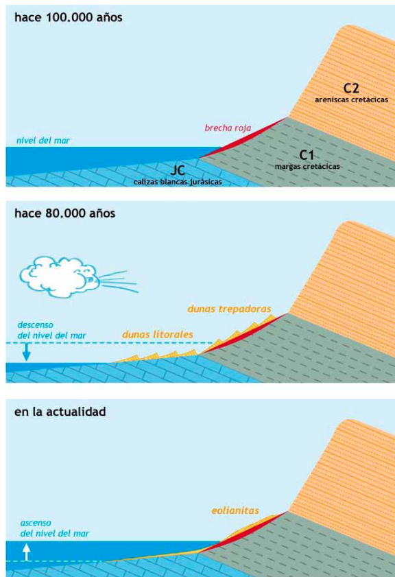
figura 11 - Esquema sobre el origen de las eolianitas
